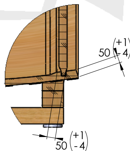
DÉTAIL G ECHELLE 1 : 14
