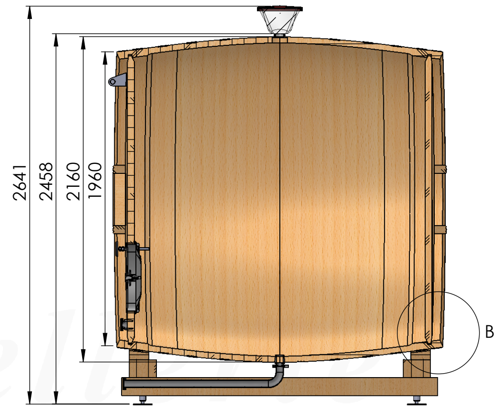
COUPE A-A
