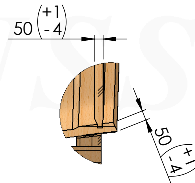
DÉTAIL B ECHELLE 1 : 20
