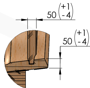
DÉTAIL B ECHELLE 1 : 10
