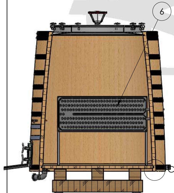
COUPE A-A ECHELLE 1 : 30
