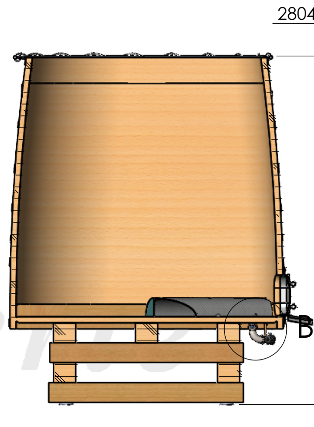
COUPE A-A ECHELLE 1 : 30
