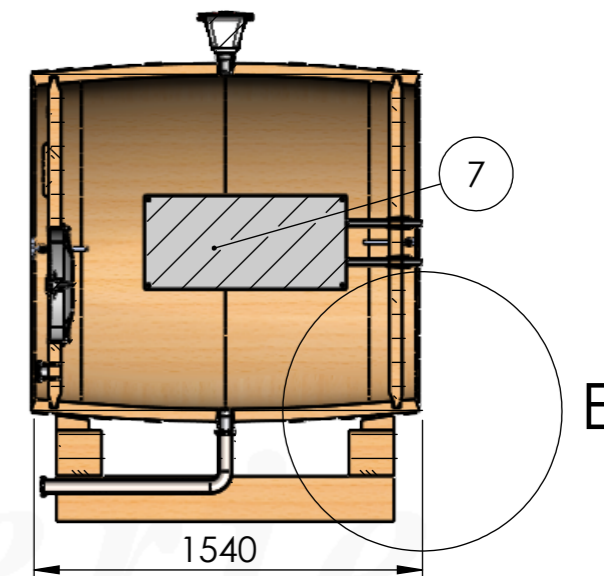
COUPE D-D ECHELLE 1 : 30
