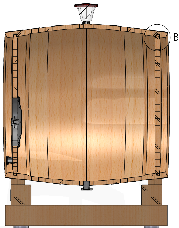
COUPE A-A ECHELLE 1 : 20
