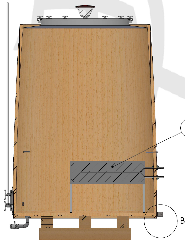
COUPE A-A ECHELLE 1 : 30
