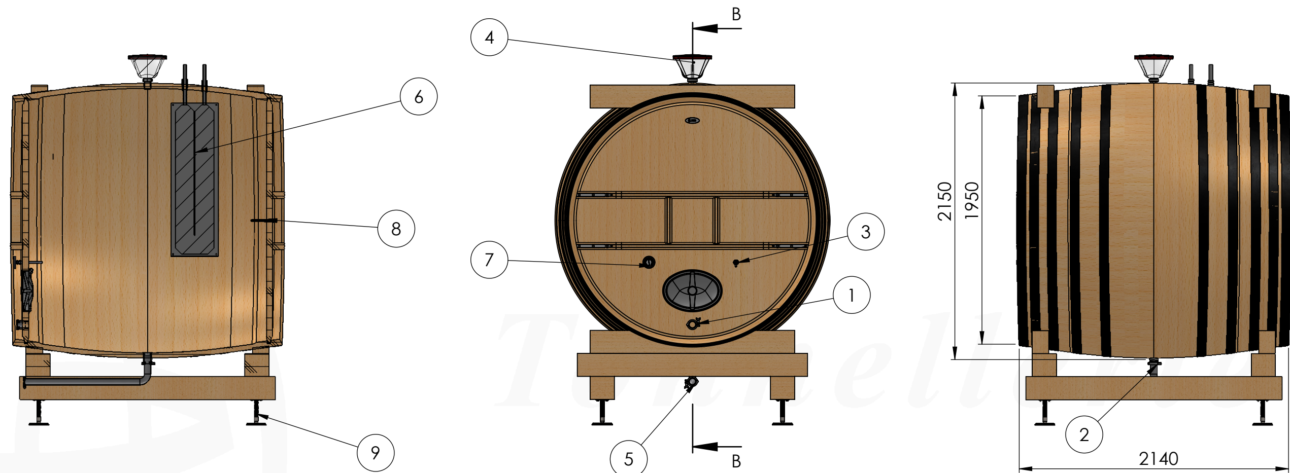
COUPE B-B
